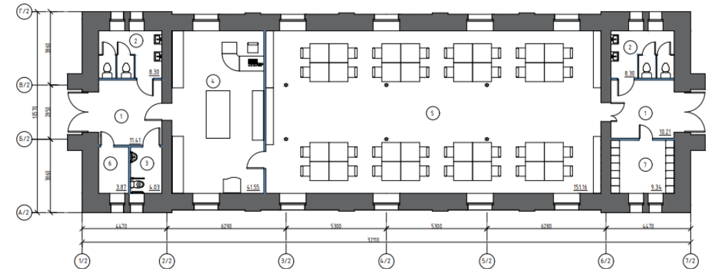
План 1-го этажа кожевенной мастерской
