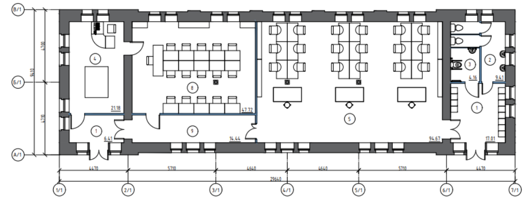
План 1-го этажа ювелирной мастерской
